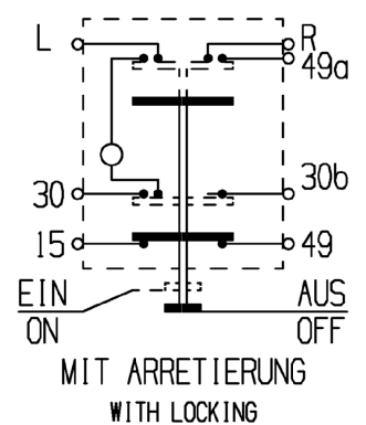
Schaltbild
