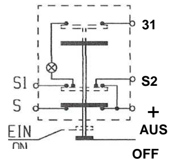
Schaltbild
