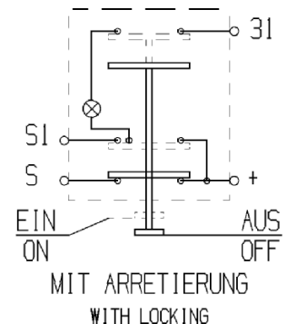
Schaltbild
