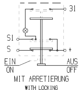
Schaltbild
