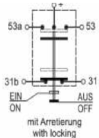
Schaltbild
