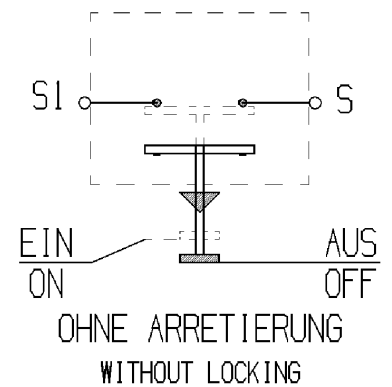
Schaltbild
