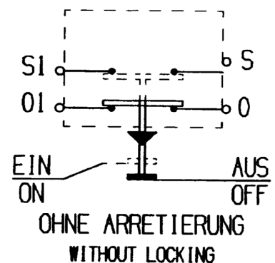
Schaltbild
