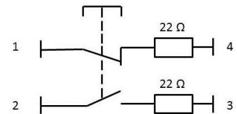
Schaltbild
