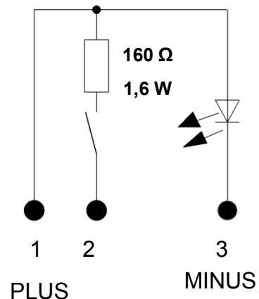
Schaltbild
