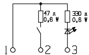
Schaltbild
